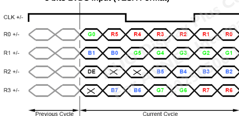
8 bits LVDS Input (VESA Format)
