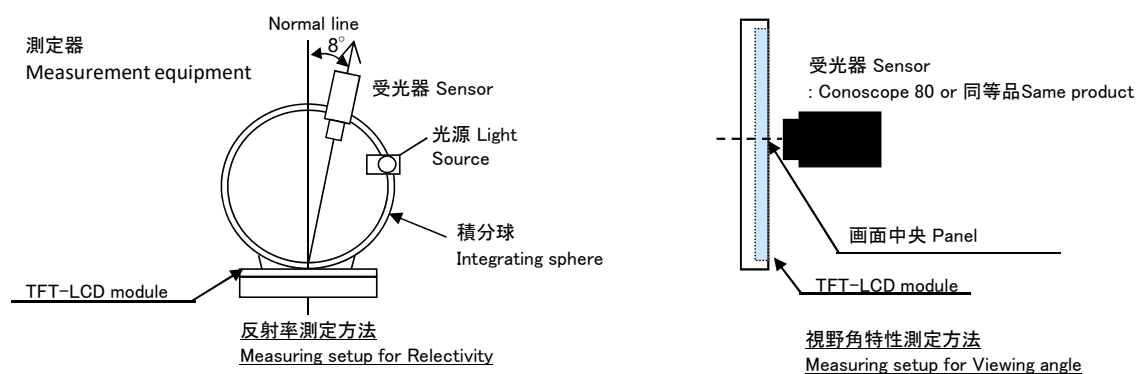
図2-1 光学的特性測定方法(反射) Optical characteristics measurement method
