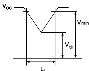
瞬時電圧降下 V CC -dip conditions
