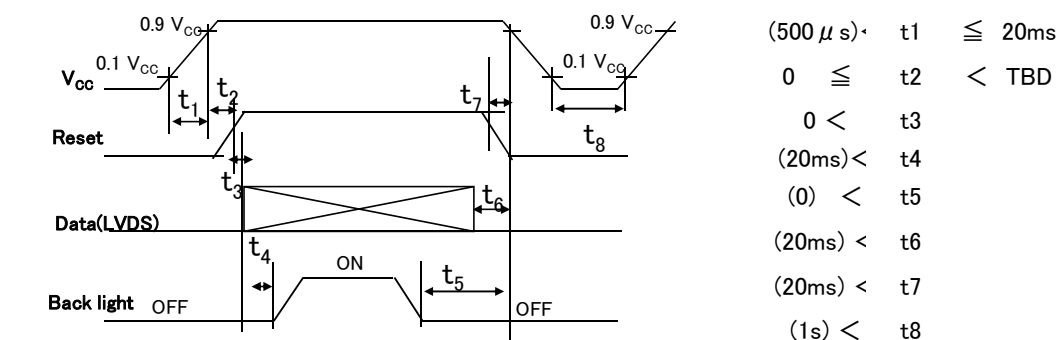
瞬時電圧降下 V CC -dip conditions
