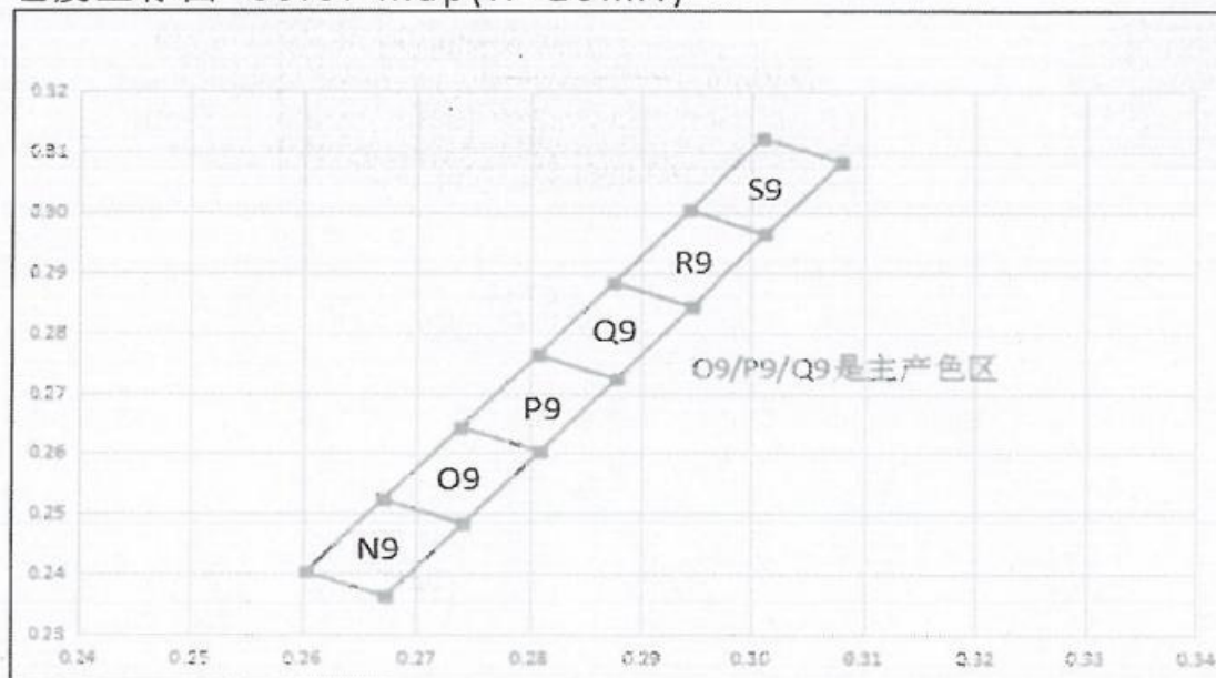
色度坐标图 Color map(If=20mA)
